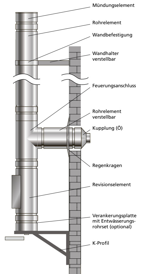
Montage am Gebäude mit K-Profilen und Wandhaltern
