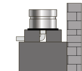
Montage am Gebäude auf tragfähigem Fundament
