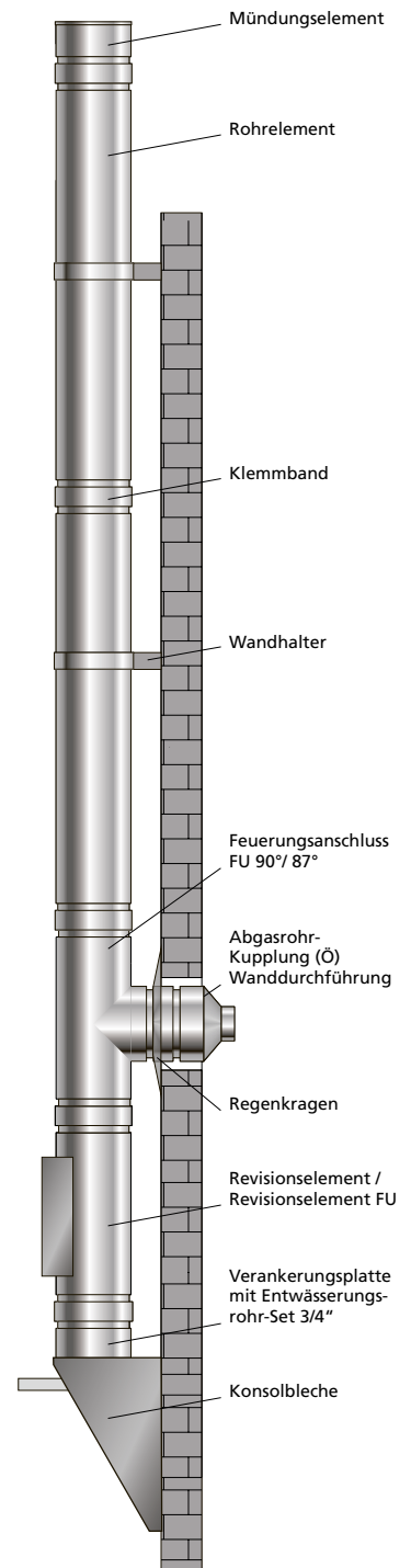
Montage am Gebäude auf Konsolblechen
